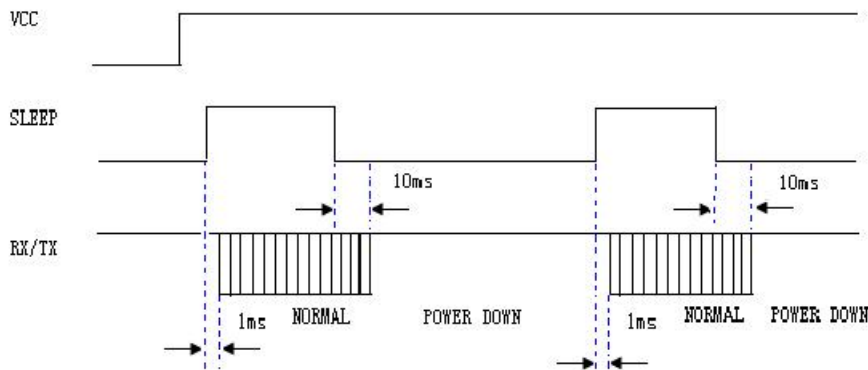
图 3：休眠时序图
