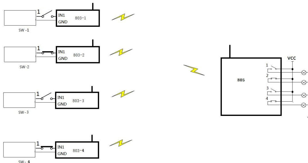
图八：4只803控制1只805
